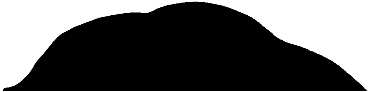
lava dome
